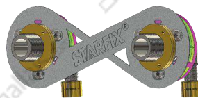
SORTIE COUDÉE M 3/4"
