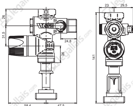
NA53M2 - modèle droit
