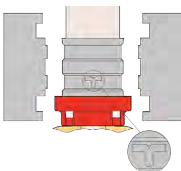
Illustration du logo imprimé sur la bague après l'opération de sertissage effectuée avec pince profil TH - personnalisée Tiemme
