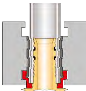
Profil pince : TH - personnalisé Tiemme Profil pince : TH
