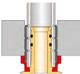
Profil pince : H
